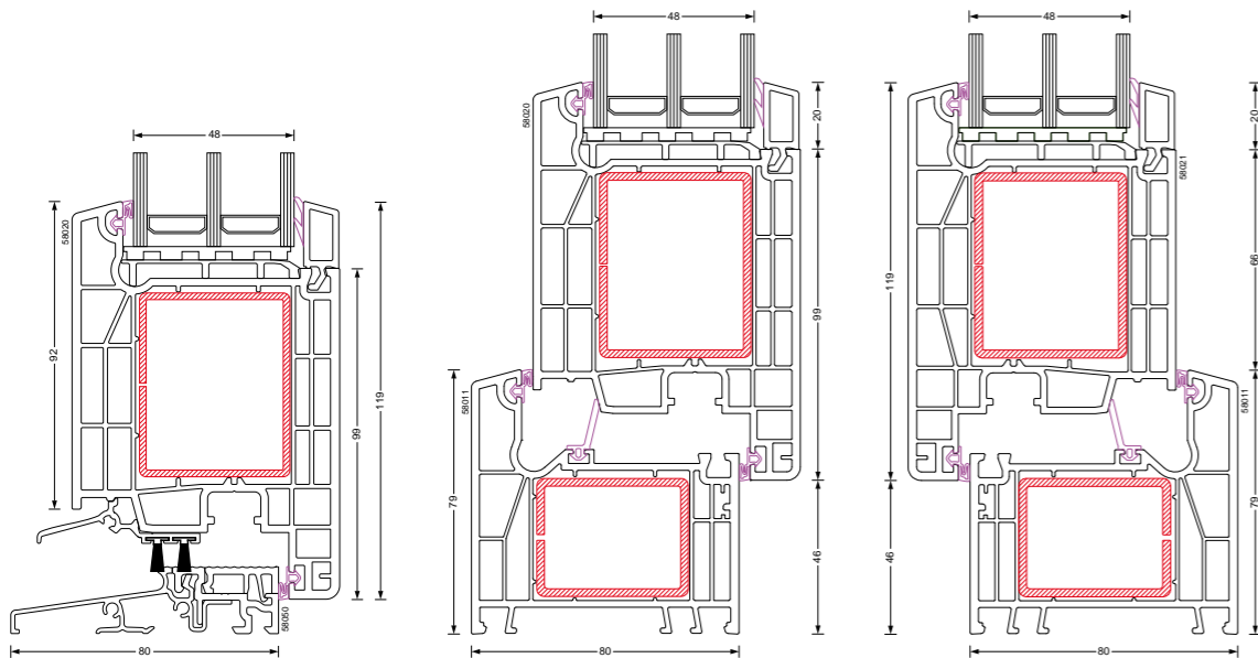
Schwelle 58050 - 58020
